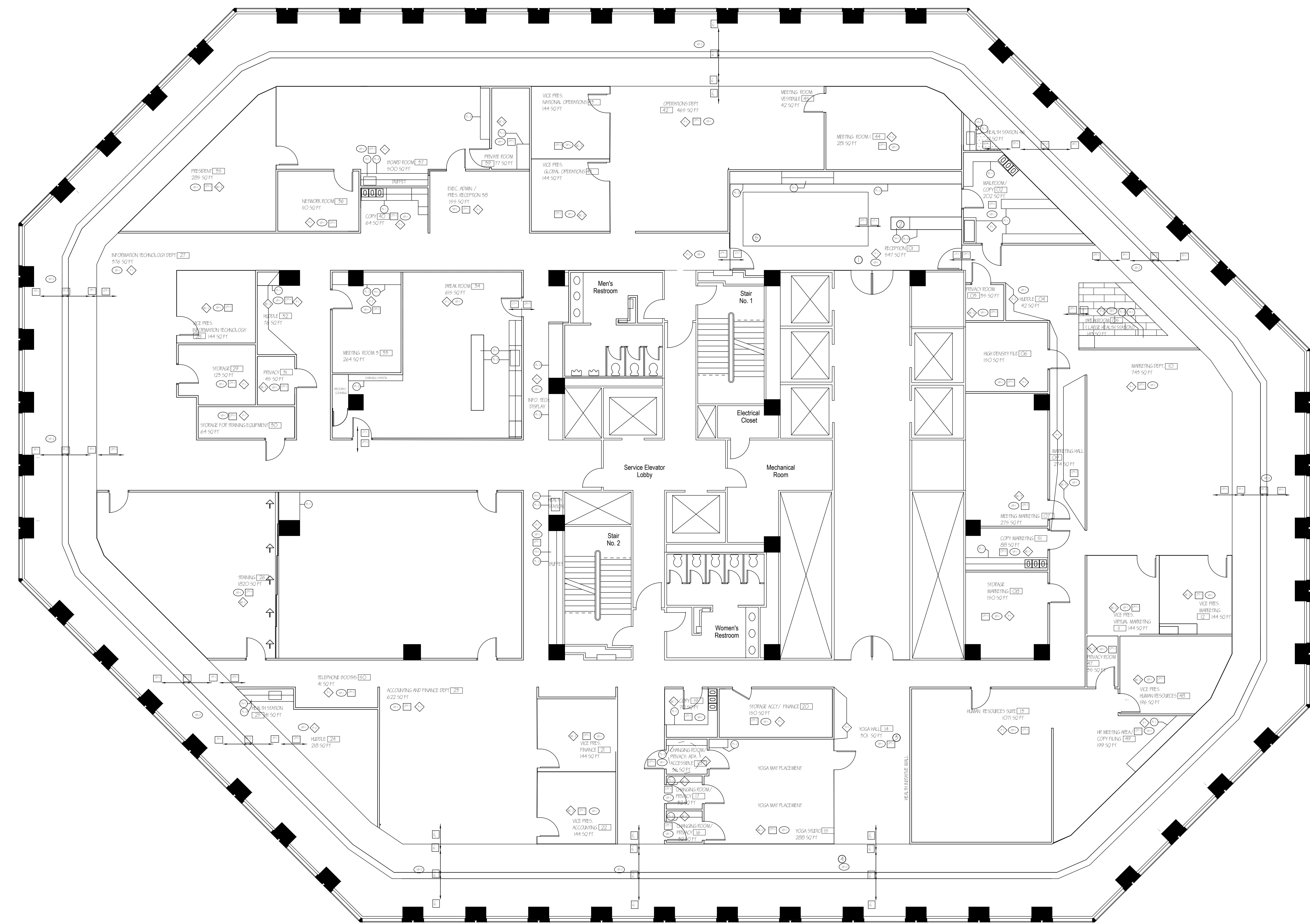
1 FINISH PLAN SCALE: 1/8" = 1'-0"
